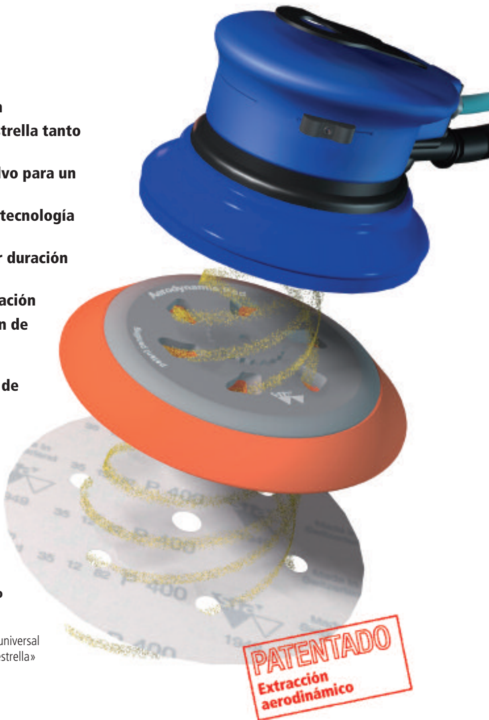
Plato aerodinámico T7207.0000.1 extra blando incl. adaptador universal con forma de «estrella» 5/16" + M8
