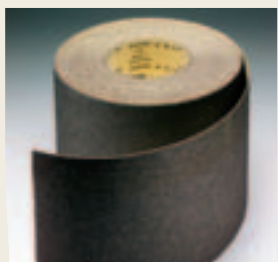
1707 siapar Rouleau série spéciale pour le ponçage de parquets, avec support adapté. Ponçage au grain grossier avec support toile coton stable, ponçage au grain moyen et fin avec support papier.
