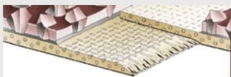
Joint à recouvrement avec enlèvement de grains
